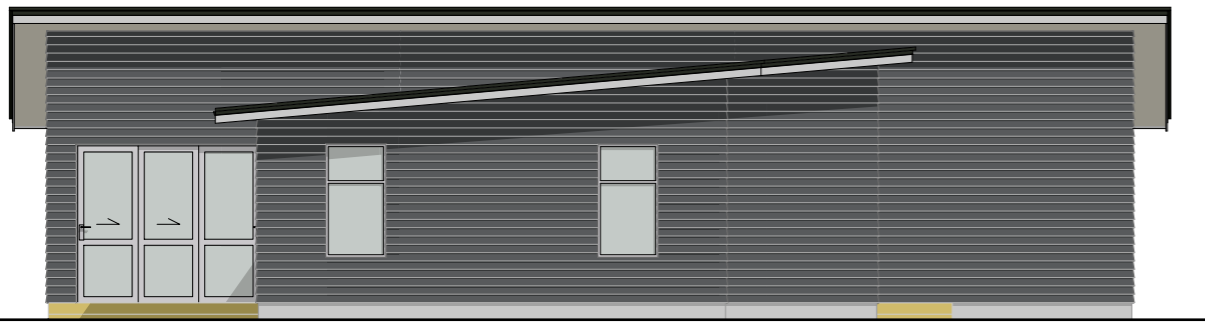
Elevation Three Scale: 1:100
