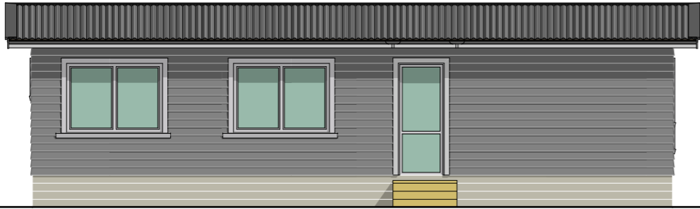
Elevation 1 Scale: 1:100
